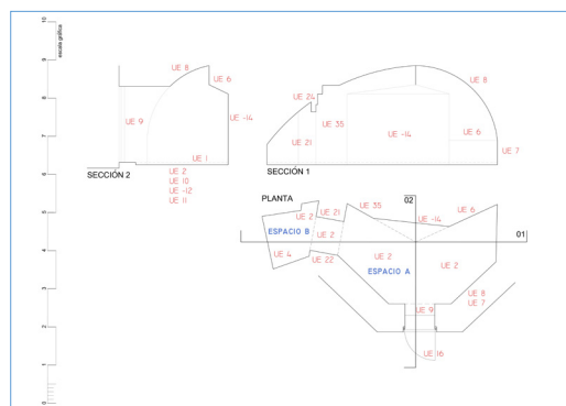
Iglesia de San Francisco, AAPre. Ubicación de las UU.EE. más significativas documentadas. Elaboración propia a partir de planimetría base de Manuel Gómez Martínez, arquitecto.
