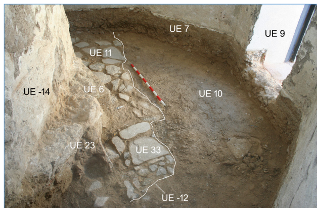
Iglesia de San Francisco, AAPre. Identificación de algunas UU.EE.
