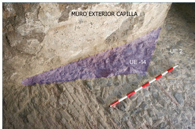
Iglesia de San Francisco, AAPre. Retallado (UE 14) del muro exterior de la capilla y relación estratigráfica con el pavimento UE 2.
