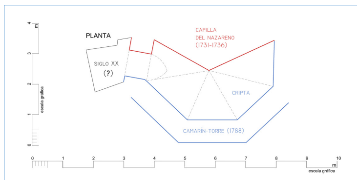
Iglesia de San Francisco, AAPre. Interpretación final del espacio barroco documentado, con camarín-torre que incluye una cripta [azul] y su adosamiento a la capilla nazarena [rojo]. Elaboración propia a partir de planimetría base de Manuel Gómez Martínez, arquitecto.
